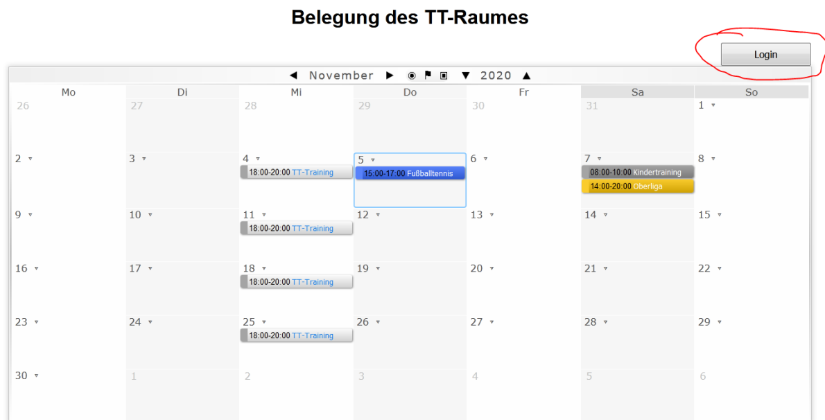
Abbildung 1: Kalenderübersicht
